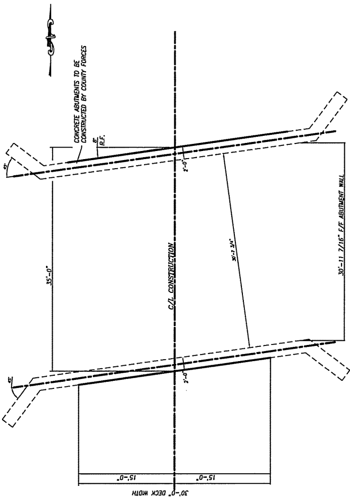
STRUCTURE SC 32-0.19 N.T.S.
